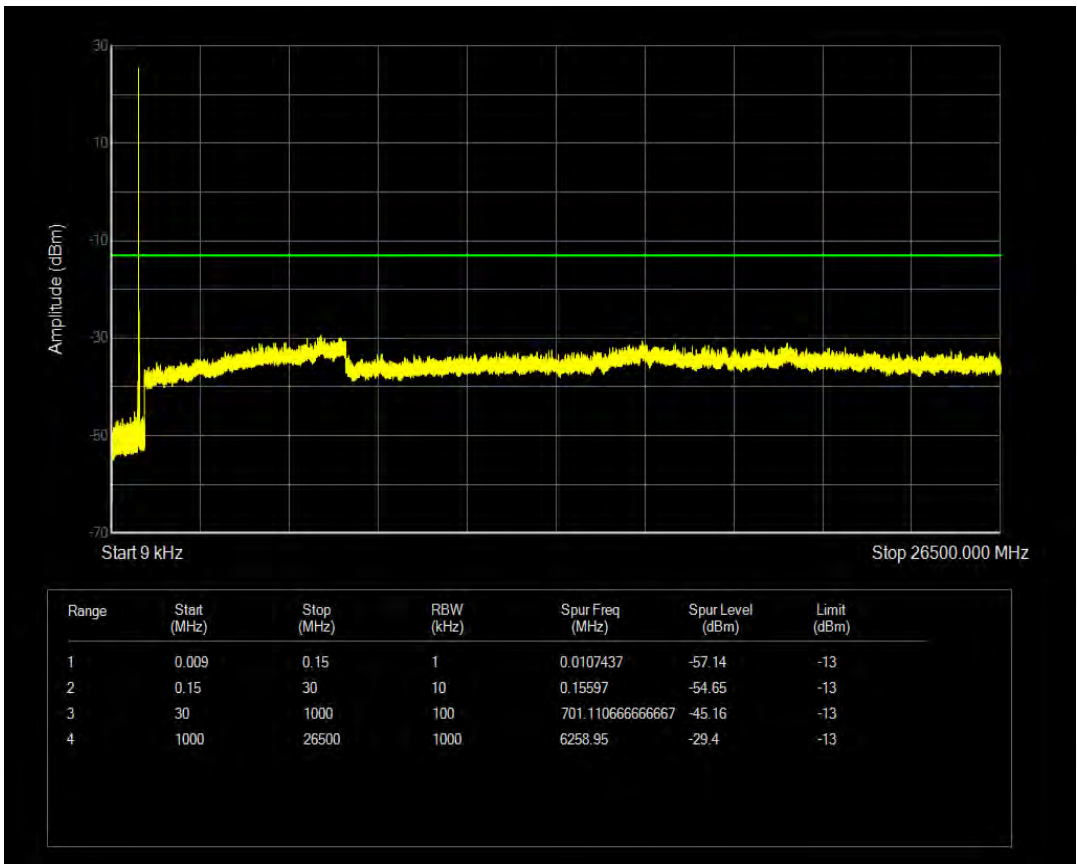
n5 SCS=15kHz CP_QPSK BW=25MHz Channel=167300 RB=1@132
