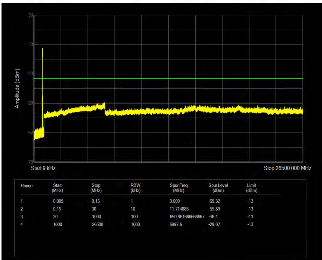
n5 SCS=15kHz CP_QPSK BW=25MHz Channel=167300 RB=1@0
