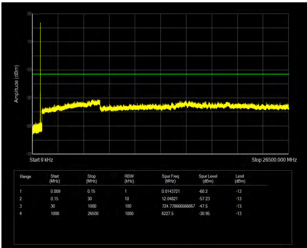
n5 SCS=15kHz CP_QPSK BW=25MHz Channel=167300 RB=133@0
