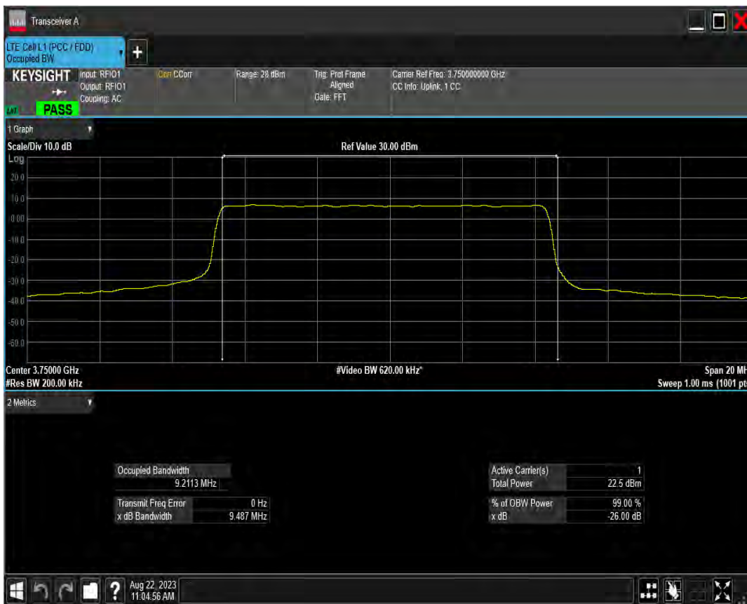
n78(3700-3800) SCS=15kHz DFT 16QAM BW=10MHz Channel=653000 RB=50@0
