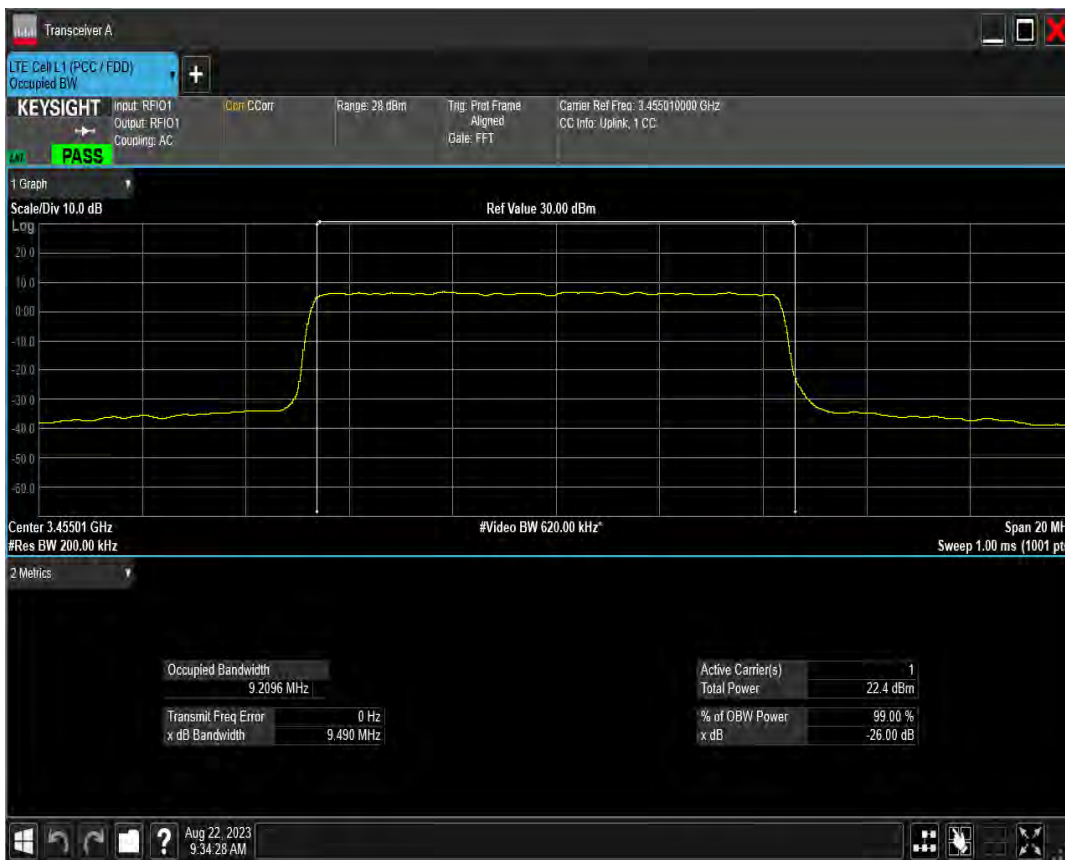
n78(3450-3550) SCS=15kHz DFT 64QAM BW=10MHz Channel=633334 RB=50@0
