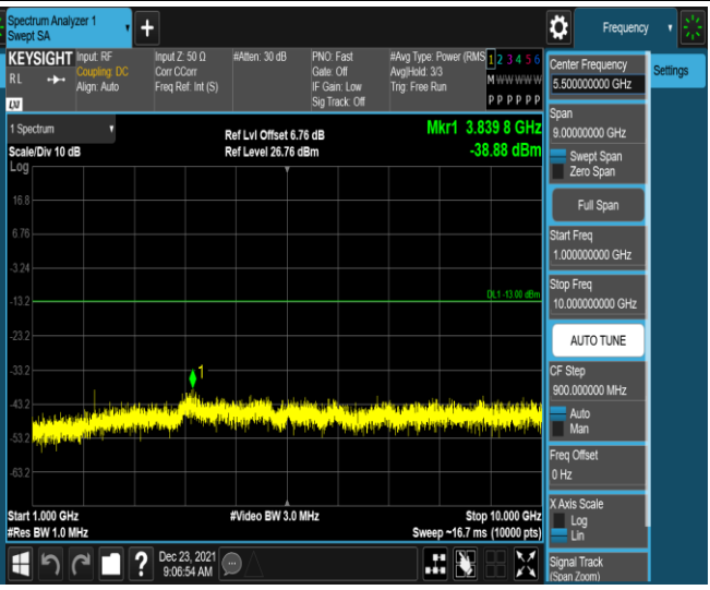
Band12-10MHz-QPSK-23060-1RB#0-Range2:1000~ 0000MHz
