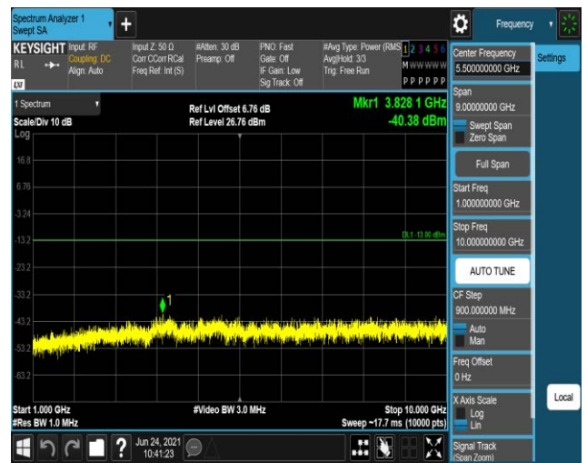
Band12-1.4MHz-QPSK-23095:1000~10000MHz
