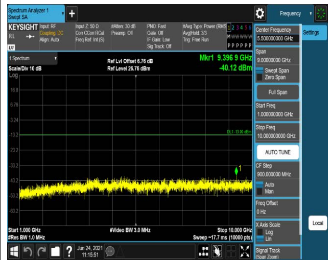
Band12-10MHz-QPSK-23095:1000~10000MHz
