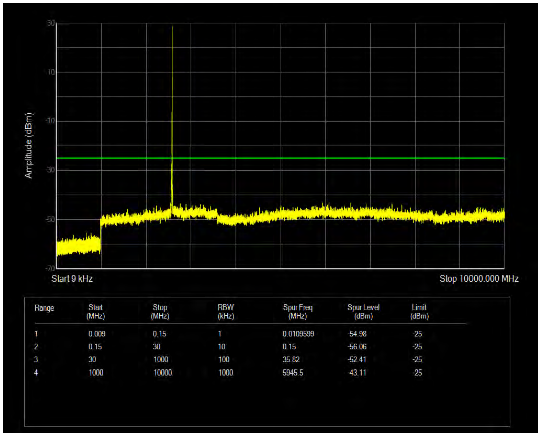
n41 SCS=30kHz CP_QPSK BW=10MHz Channel=537000 RB=24@0
