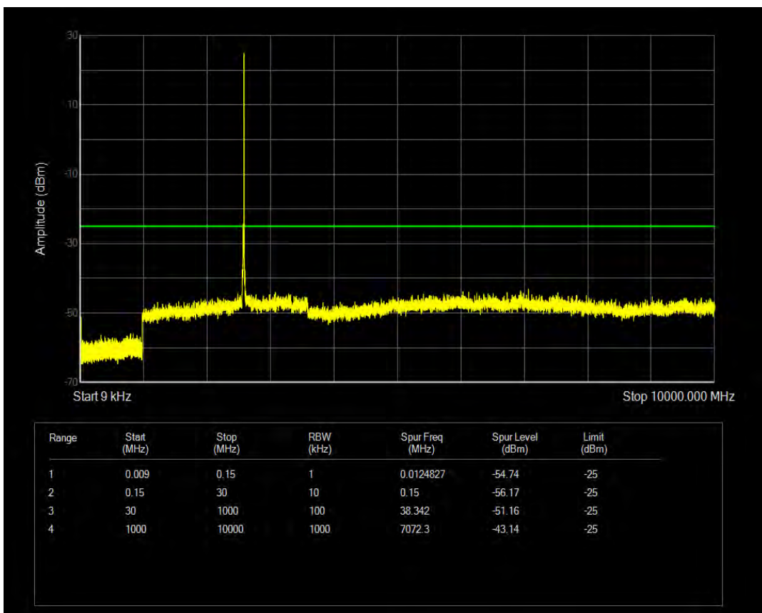
n41 SCS=30kHz CP_QPSK BW=15MHz Channel=536496 RB=38@0
