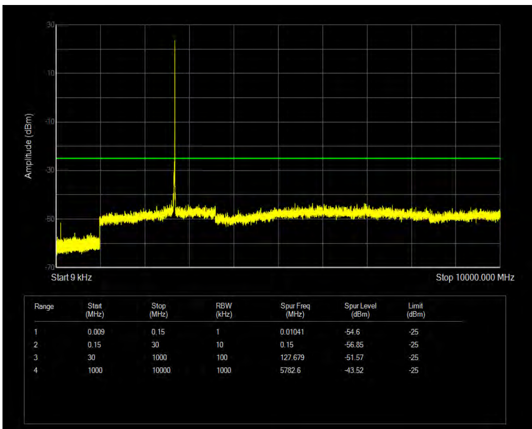
n41 SCS=30kHz CP_QPSK BW=40MHz Channel=503202 RB=106@0
