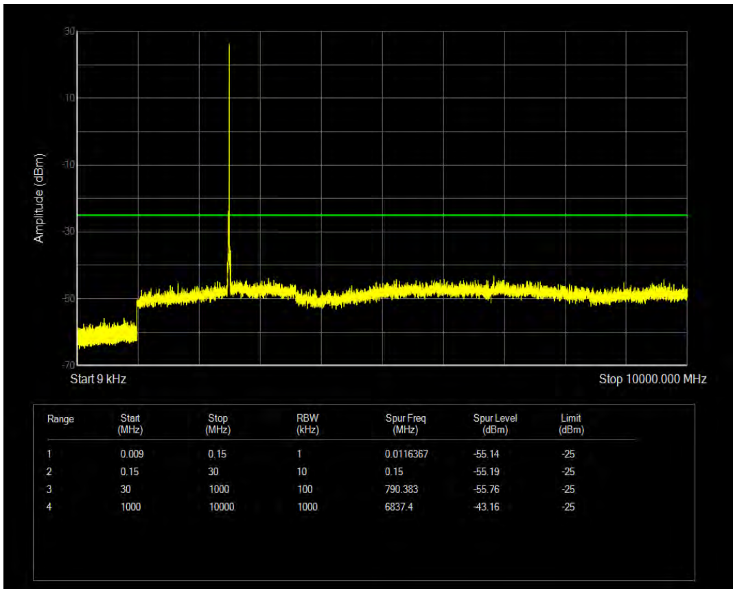
n41 SCS=30kHz CP_QPSK BW=15MHz Channel=518598 RB=38@0
