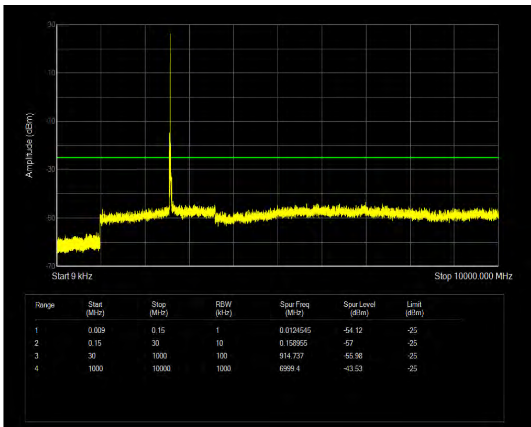
n41 SCS=30kHz CP_QPSK BW=20MHz Channel=518598 RB=1 @50
