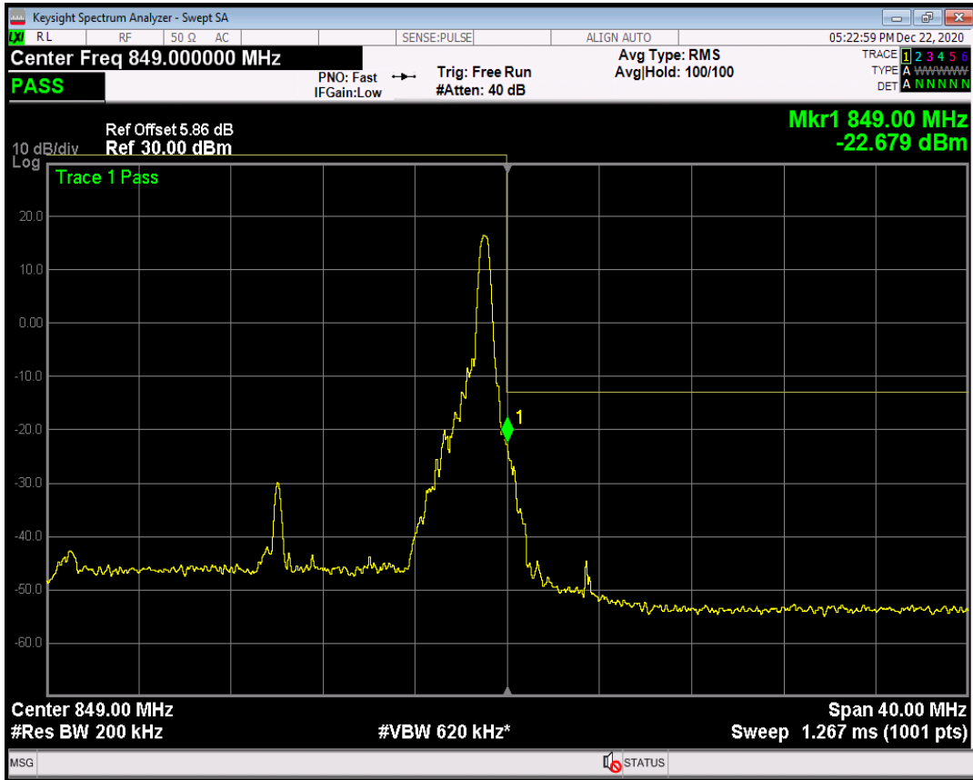
n5 SCS=30kHz CP_QPSK BW=20MHz Channel=167800 RB=50@0
