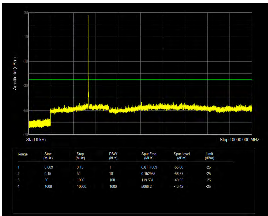
n41 SCS=30kHz CP_QPSK BW=10MHz Channel=537000 RB=1@23
