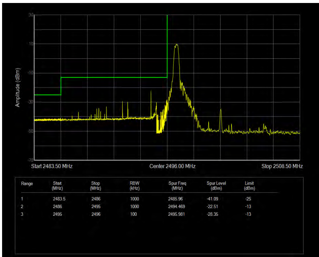
n41 SCS=30kHz CP_QPSK BW=10MHz Channel=500202 RB=1 @23
