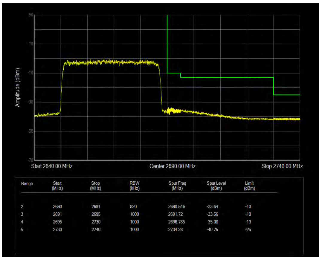
n41 SCS=30kHz CP_QPSK BW=40MHz Channel=534000 RB=1@0
