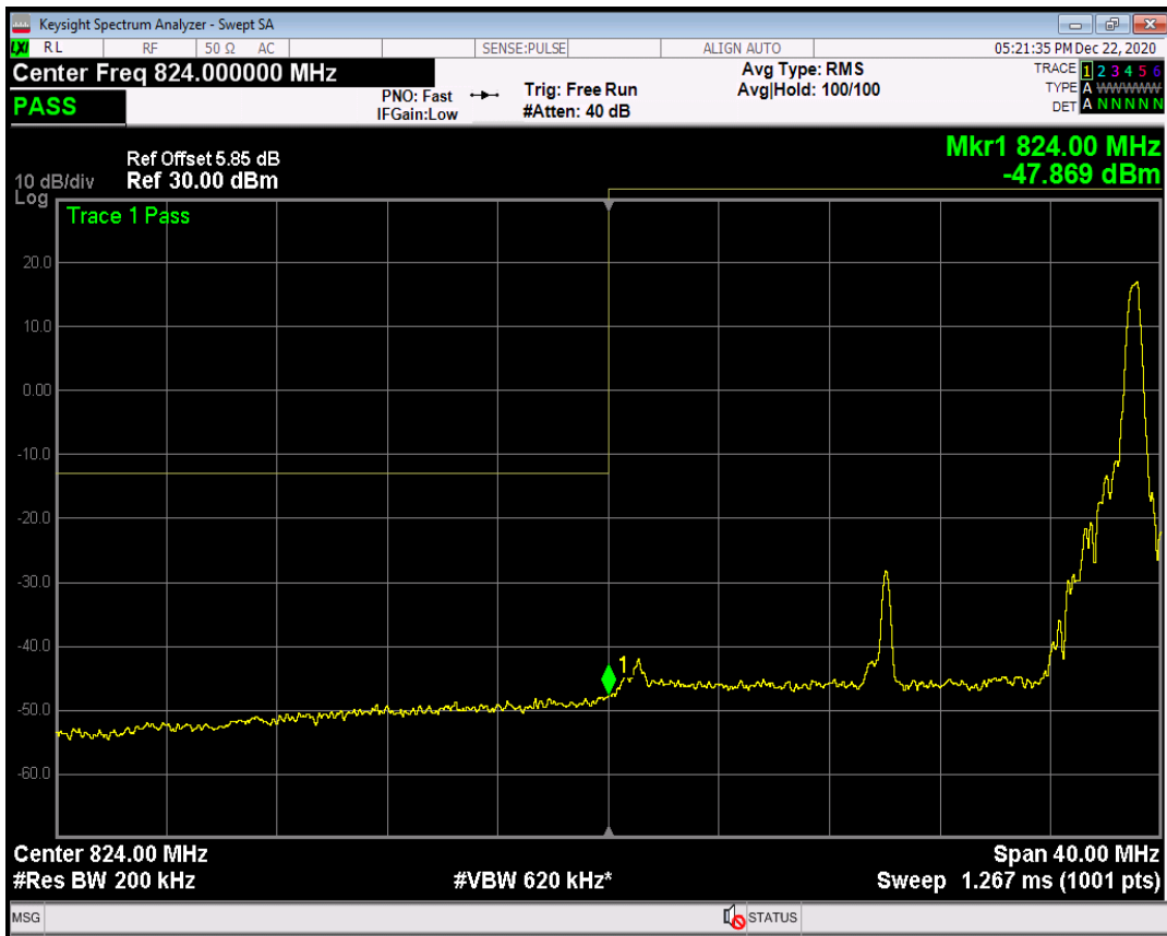
n5 SCS=30kHz CP_QPSK BW=20MHz Channel=166800 RB=50@0
