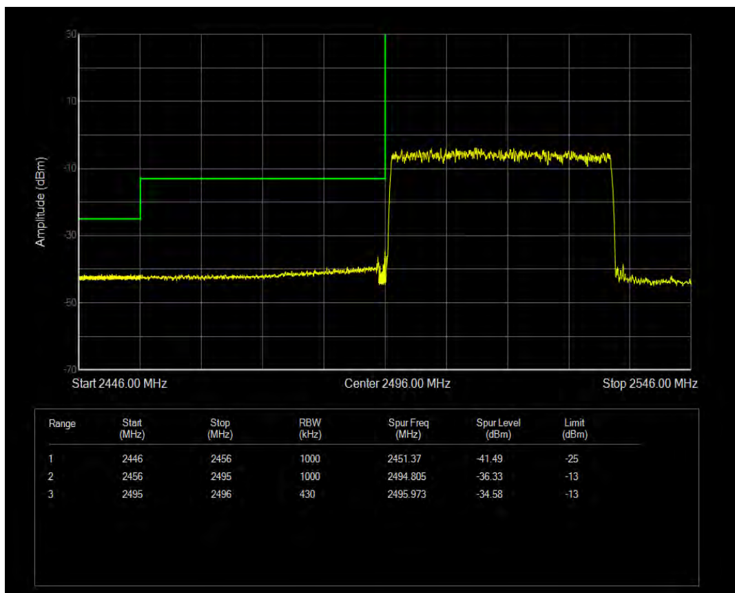
n41 SCS=30kHz CP_QPSK BW=40MHz Channel=503202 RB=1@0
