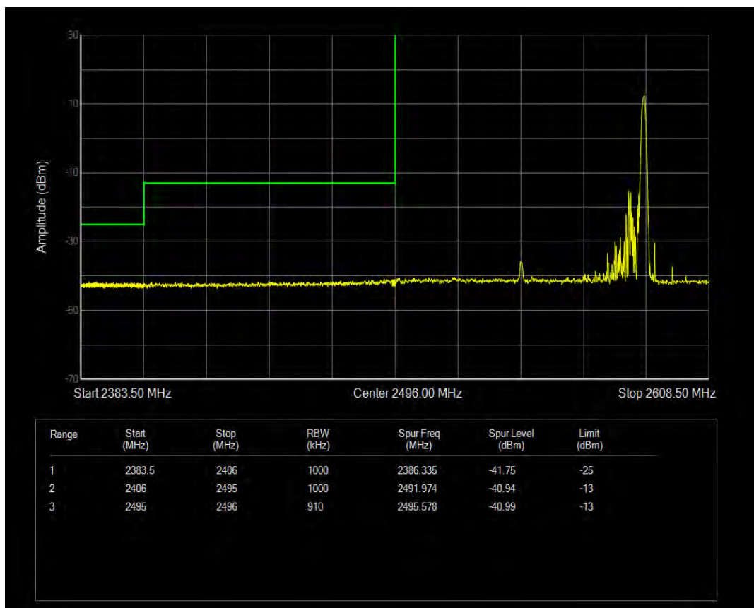
n41 SCS=30kHz CP_QPSK BW=90MHz Channel=528996 RB=240@0
