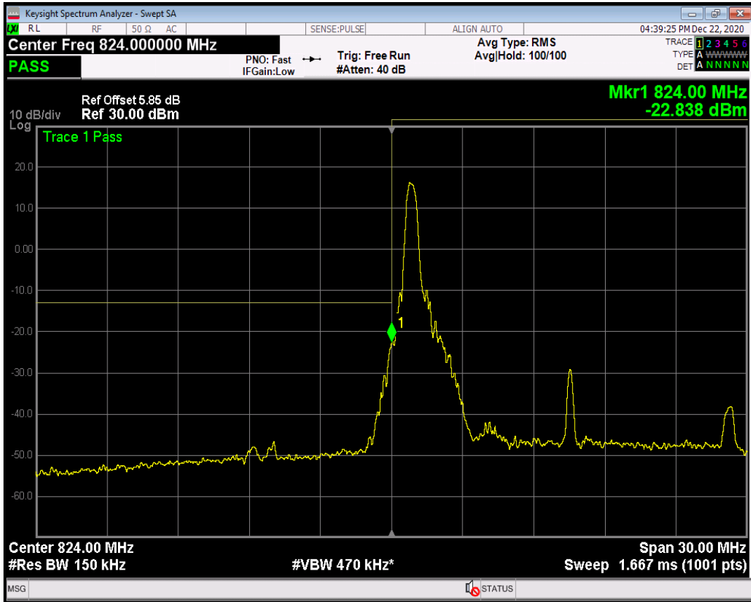
n5 SCS=30kHz CP_QPSK BW=15MHz Channel=166300 RB=1@37
