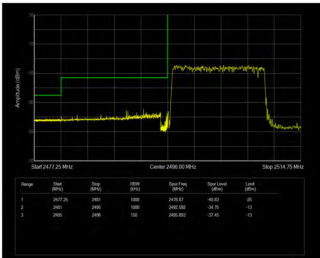
n41 SCS=30kHz CP_QPSK BW=15MHz Channel=500700 RB=1@0
