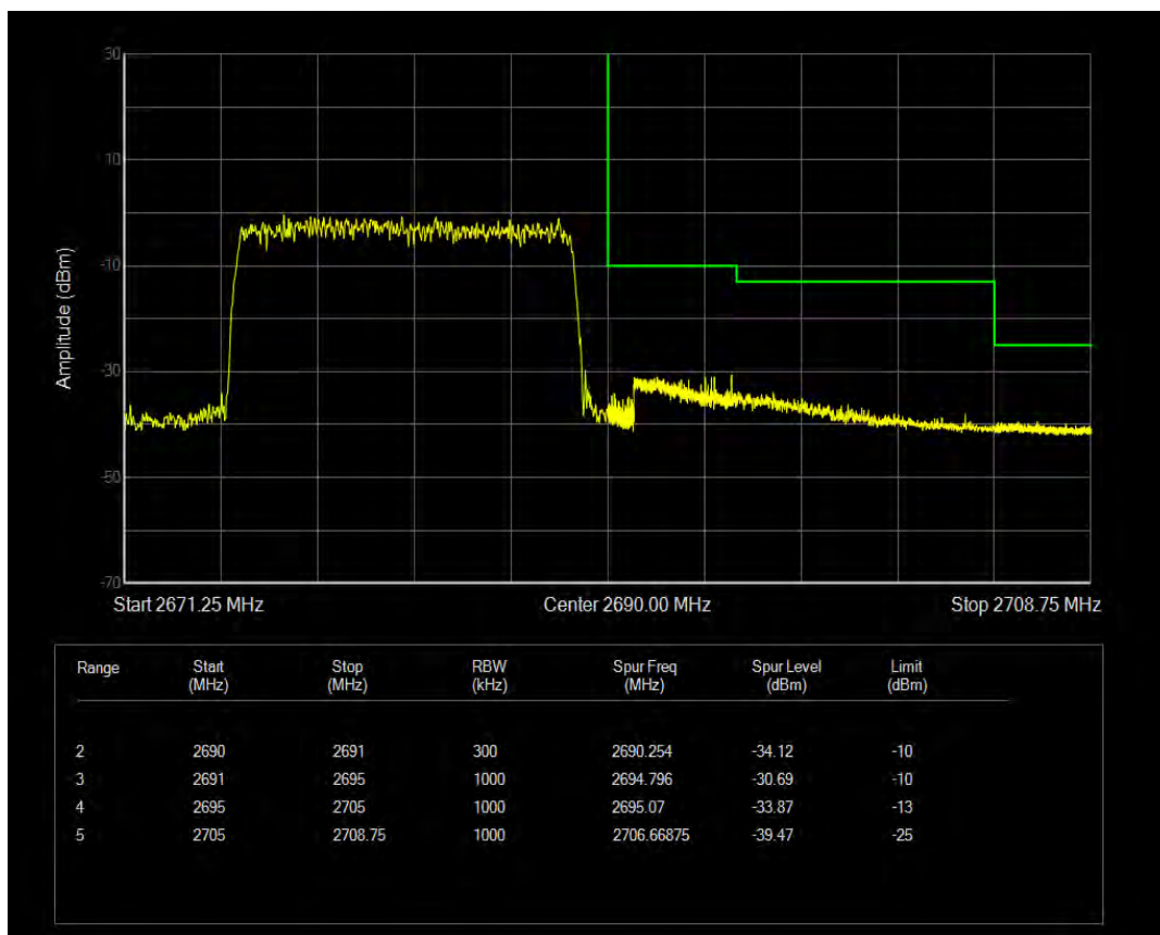
n41 SCS=30kHz CP_QPSK BW=15MHz Channel=536496 RB=1@0
