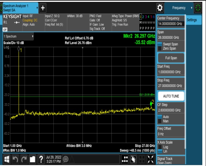
Band7-20MHz-QPSK-21350-1RB#0-Range2:1000~27000MHz
