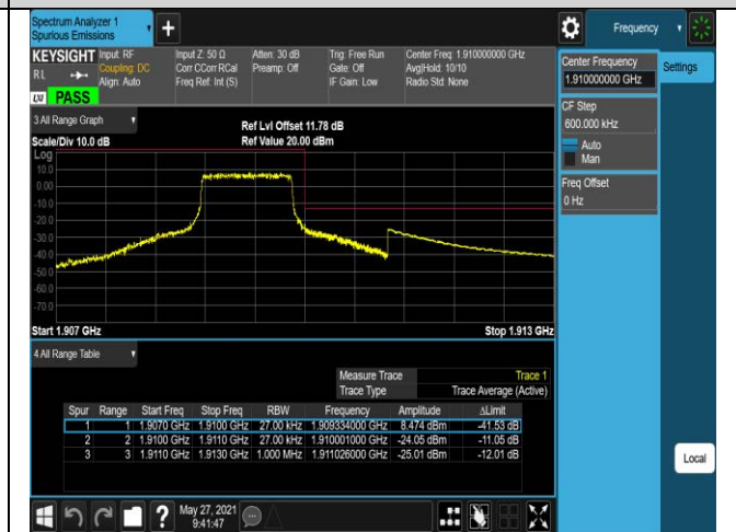
Band2-20MHz-QPSK-18700-1RB#99
