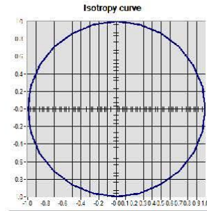
Isotropy \pm 0.25\% ( \pm 0.01 dB)
