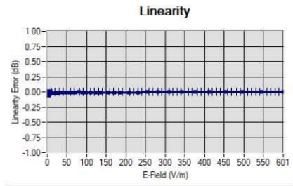
Linearity \pm 1.48\% ( \pm 0.06 dB)
