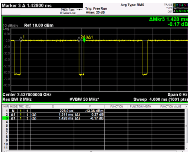
802.11n_HT20(MCS0)
