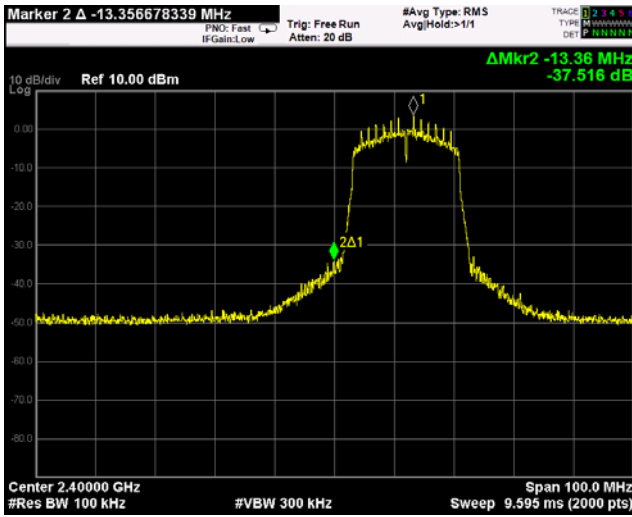
802.11n(HT40)_CH Low
