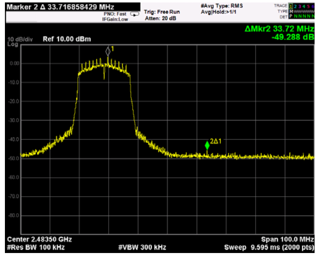
802.11n(HT40)_CH High
