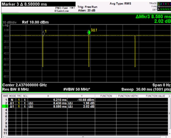
802.11n_HT20(MCS0)
