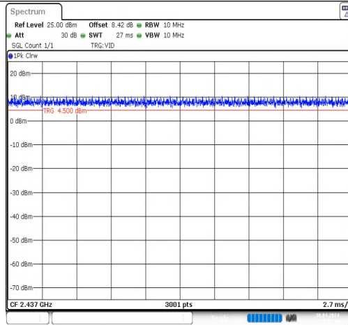
NTNV-11N20MIMO-Ant2-2437
