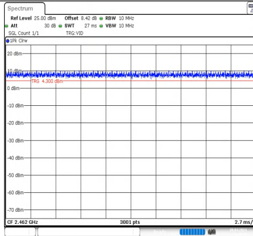
NTNV-11N20MIMO-Ant1-2462
