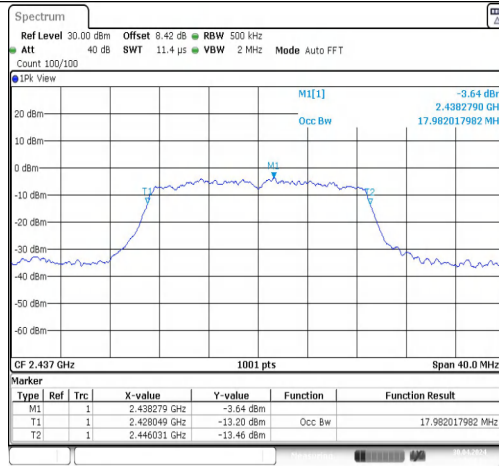
11N20MIMO-Ant2-2437
