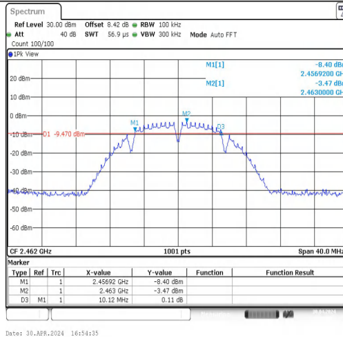
11B-CDD-Ant2-2462-PASS
