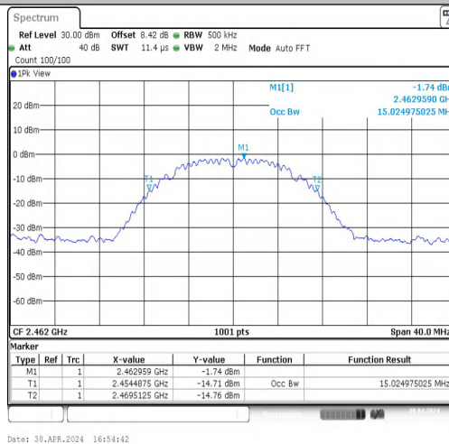
11B-CDD-Ant2-2462
