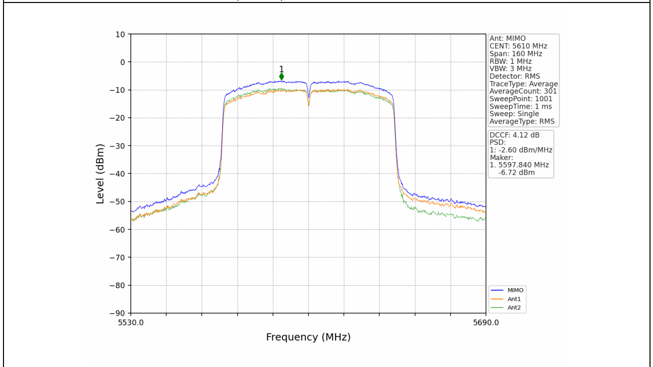
802.11ac(VHT80)_HCH_5610MHz_MIMO_NTNV
