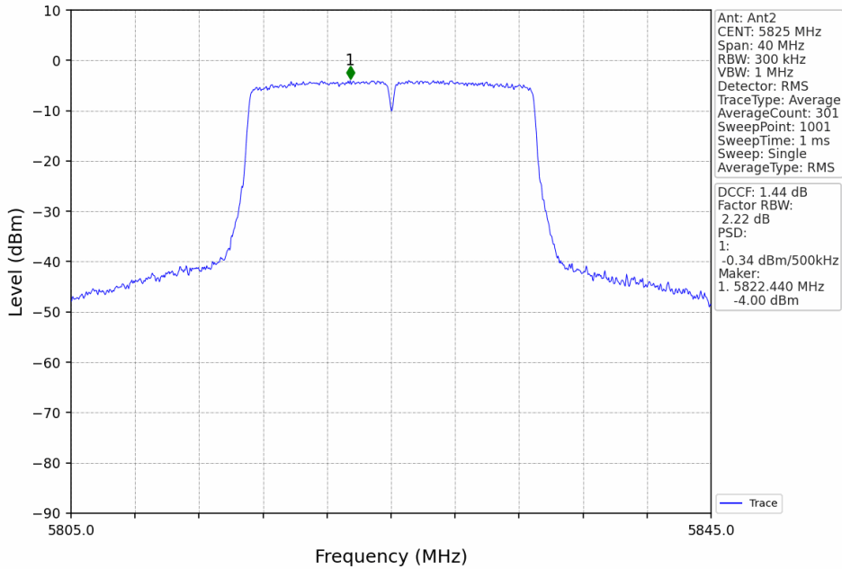
802.11n(HT20)_HCH_5825MHz_MIMO_NTNV
