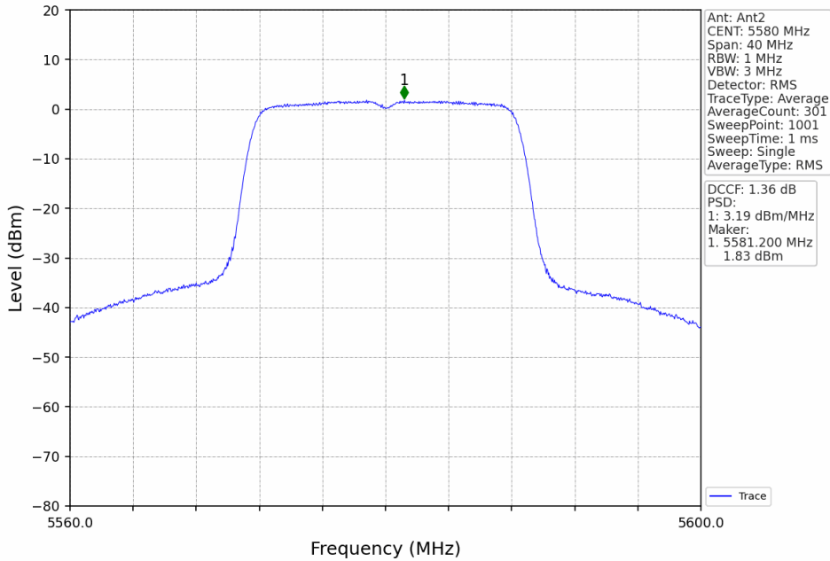
802.11a_MCH_5580MHz_MIMO_NTNV
