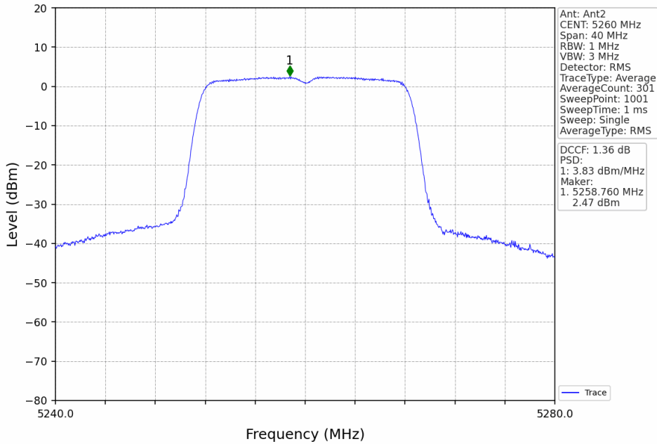
802.11a_LCH_5260MHz_MIMO_NTNV
