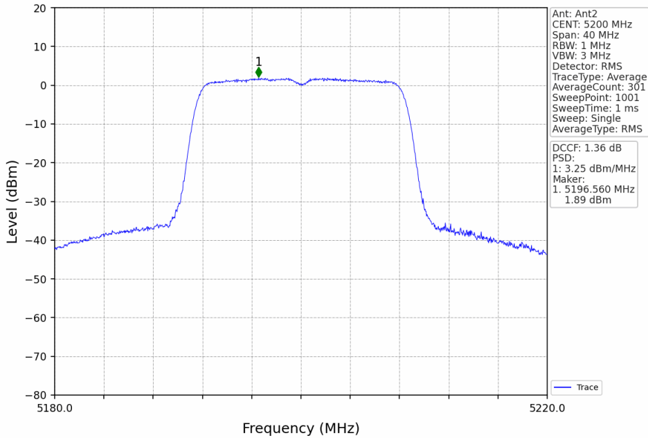
802.11a_MCH_5200MHz_MIMO_NTNV
