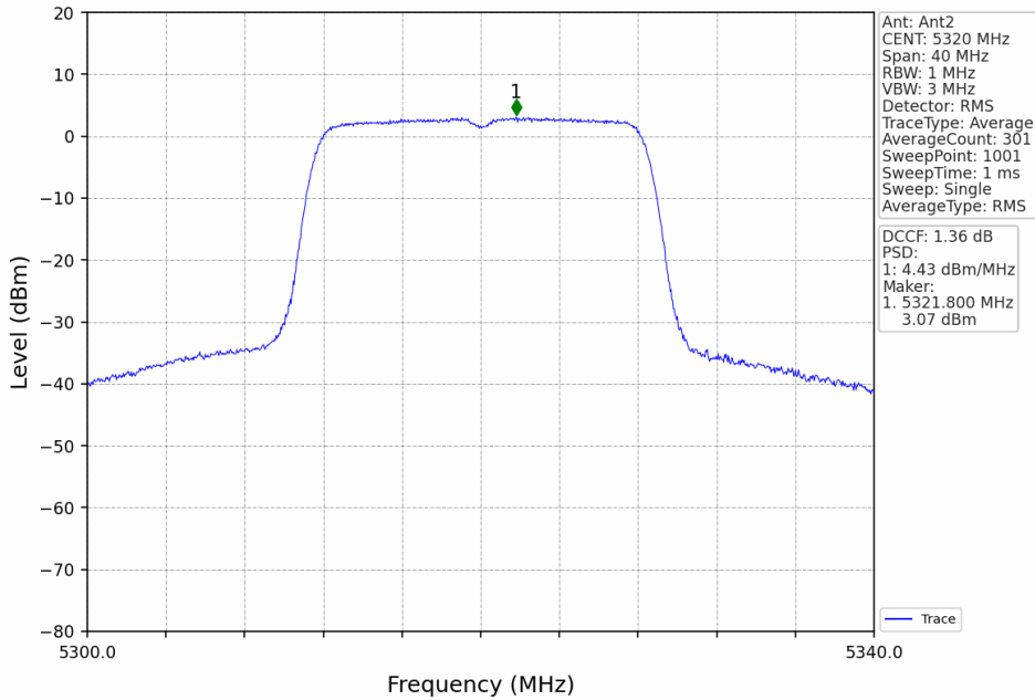
802.11a_HCH_5320MHz_MIMO_NTNV
