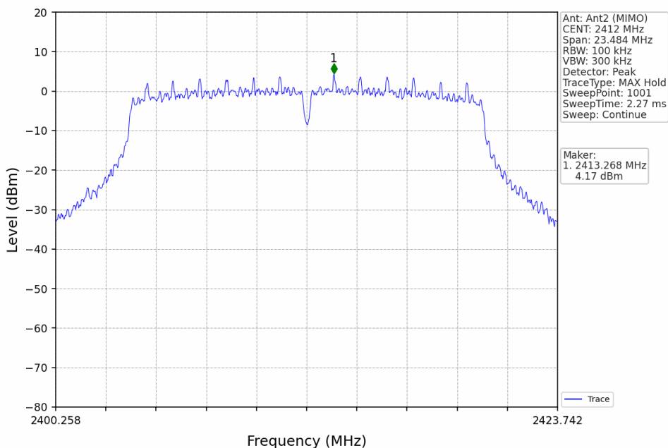
802.11g_LCH_2412MHz_Ant2 (MIMO)_NTNV
