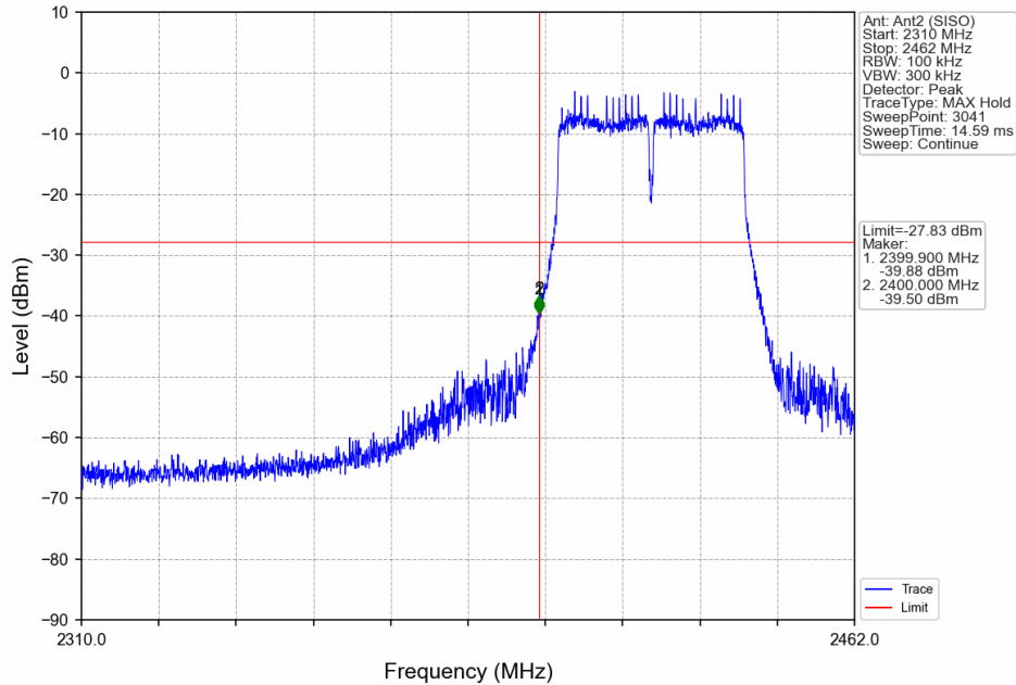
802.11n(HT40)_LCH_2422MHz_Ant2 (SISO)_NTNV
