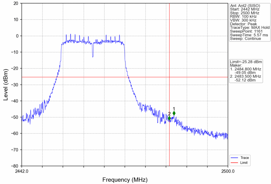
802.11n(HT20)_HCH_2462MHz_Ant2 (SISO)_NTNV
