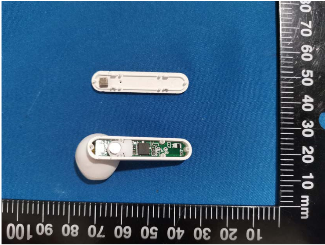
Left Unit
