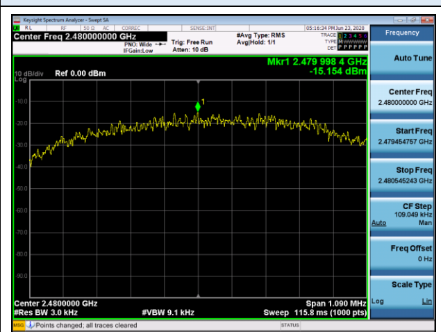
BLE 1M (MESH) : CH 39 (2480 MHz)
