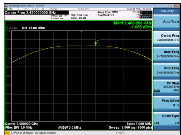
BLE 1M (MESH) : CH 39 (2480 MHz)
