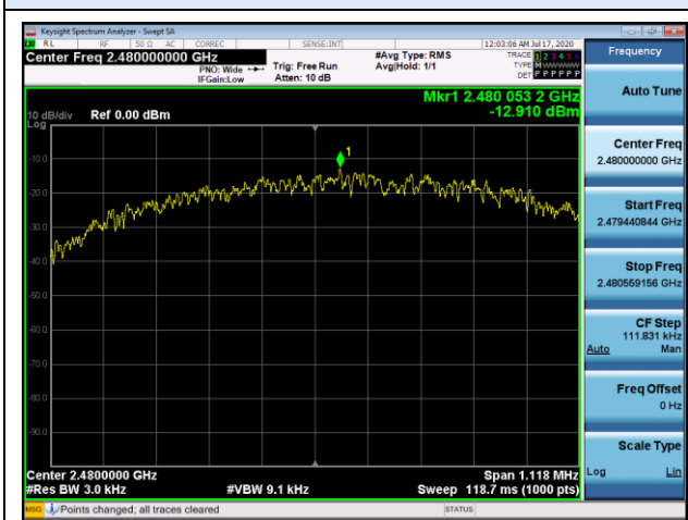
BLE 1M (MCU) : CH 39 (2480 MHz)
