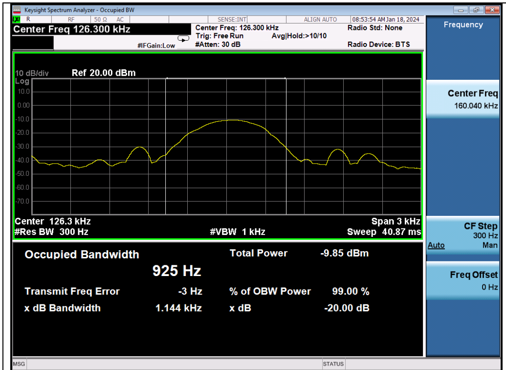
Test_Graph_ASK_Coil ANT_ 126.3kHz _ -20dB Bandwidth
