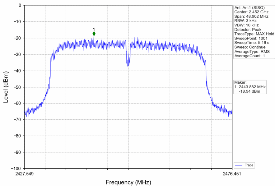
802.11n(HT40)_HCH_2452MHz_Ant1 (SISO)_NTNV
