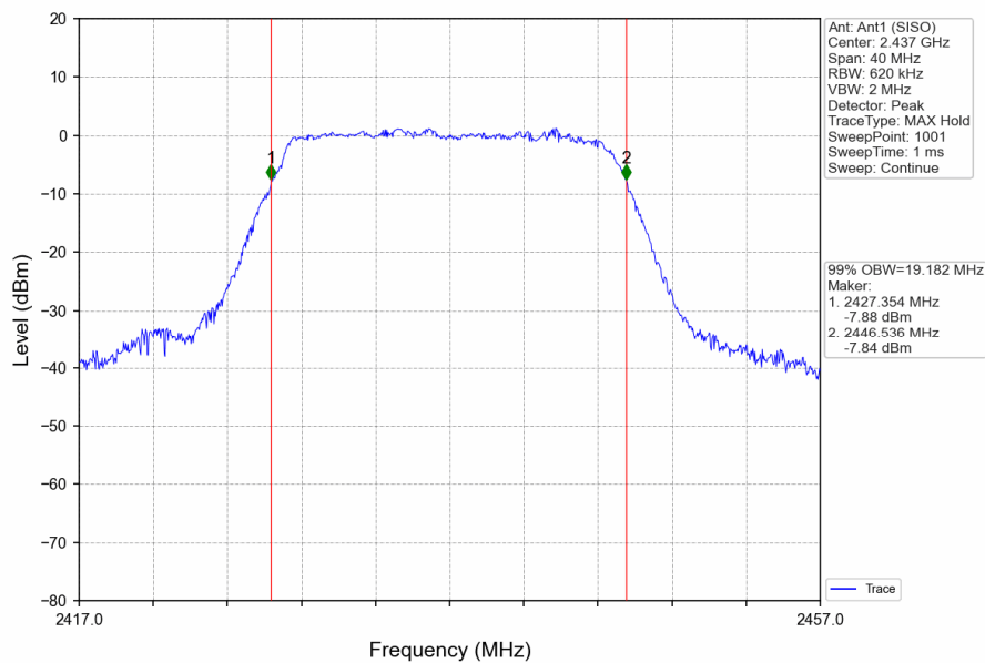
802.11n(HT20)_MCH_2437MHz_Ant1 (SISO)_NTNV
