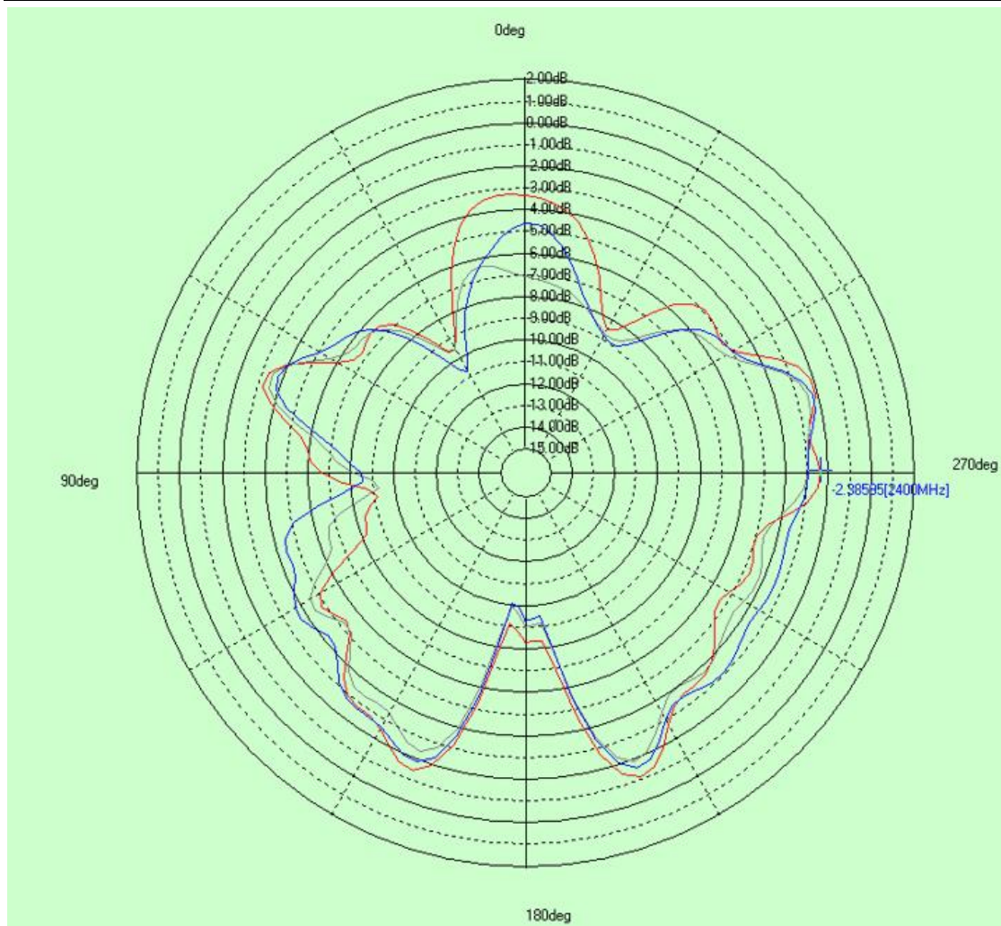
俯仰面 \phi=90^\circ
