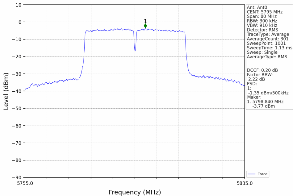
802.11ax(HEW40)_HCH_5795MHz_RU484_Left_Ant0_NTNV
