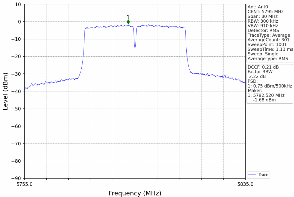
802.11ac(VHT40)_HCH_5795MHz_Ant0_NTNV
