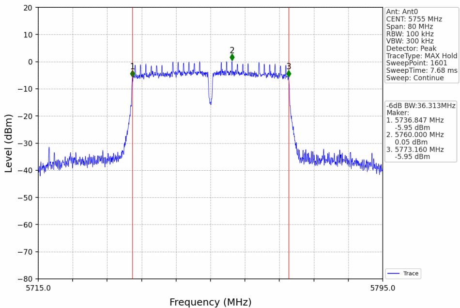
802.11ac(VHT40)_LCH_5755MHz_Ant0_NTNV
