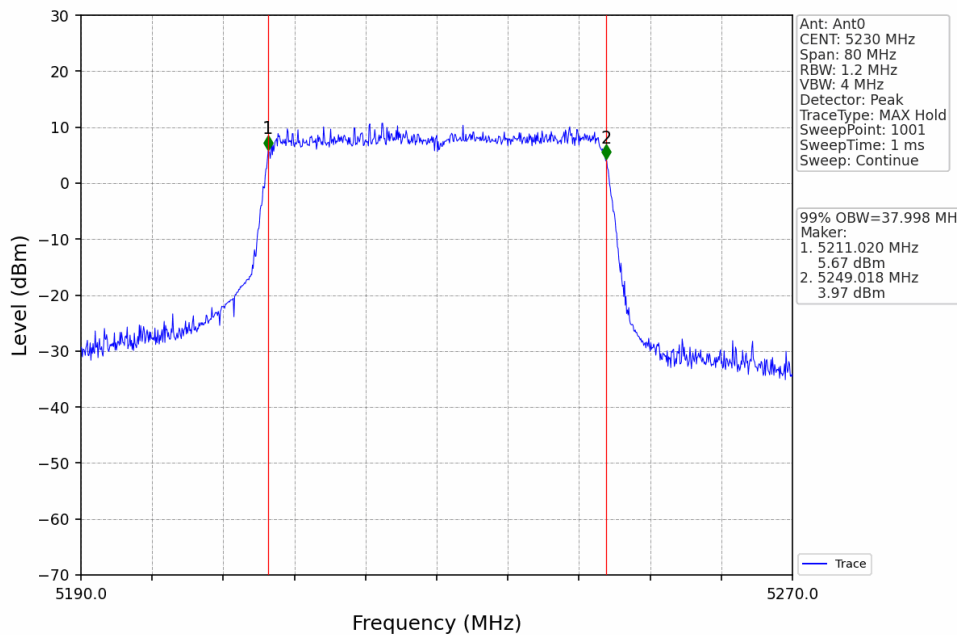
802.11ax(HEW40)_HCH_5230MHz_RU484_Left_Ant0_NTNV
