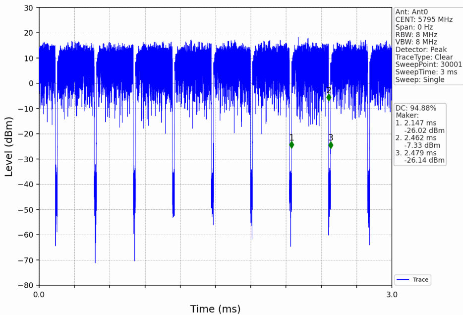
802.11ax(HEW40)_HCH_5795MHz_RU484_Left_Ant0_NTNV
