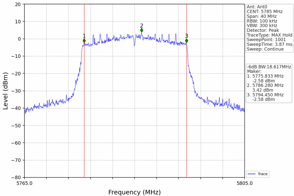
802.11ax(HEW20)_MCH_5785MHz_RU242_Left_Ant0_NTNV
