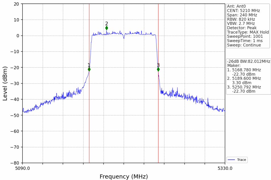
802.11ac(VHT80)_MCH_5210MHz_Ant0_NTNV
