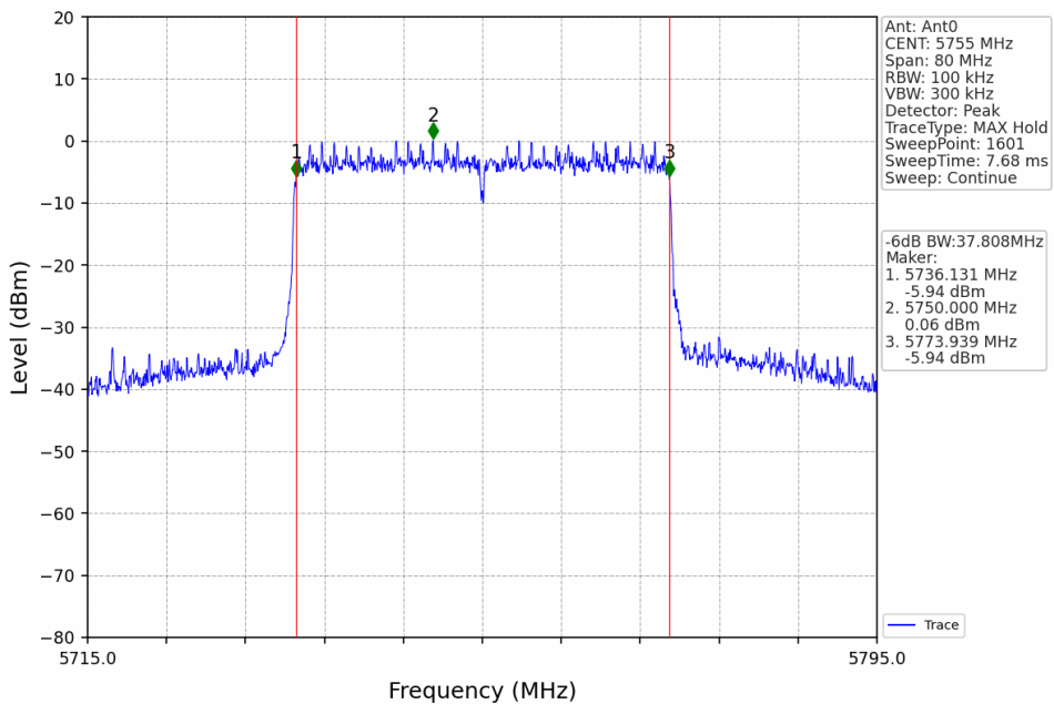
802.11ax(HEW40)_LCH_5755MHz_RU484_Left_Ant0_NTNV
