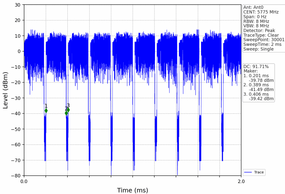
802.11ax(HEW80)_MCH_5775MHz_RU996_Left_Ant0_NTNV
