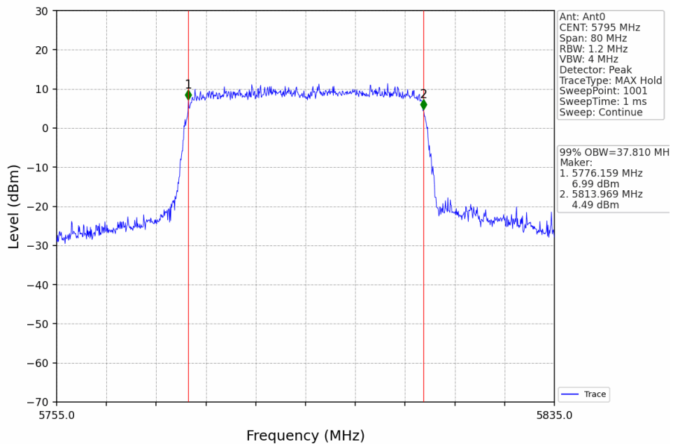
802.11ax(HEW40)_HCH_5795MHz_RU484_Left_Ant0_NTNV
