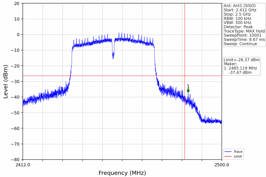
802.11n(HT40)_HCH_2452MHz_Ant1 (SISO)_NTNV
