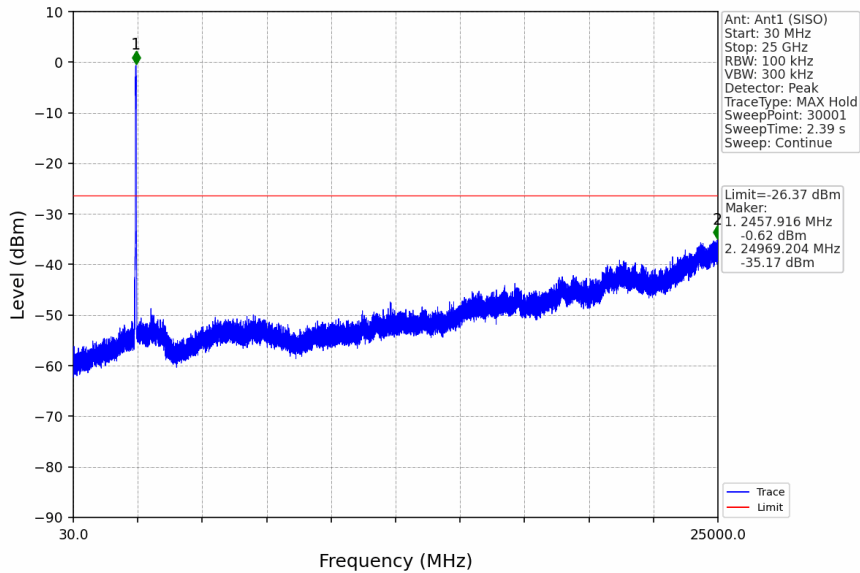
802.11n(HT40)_HCH_2452MHz_Ant1 (SISO)_NTNV
