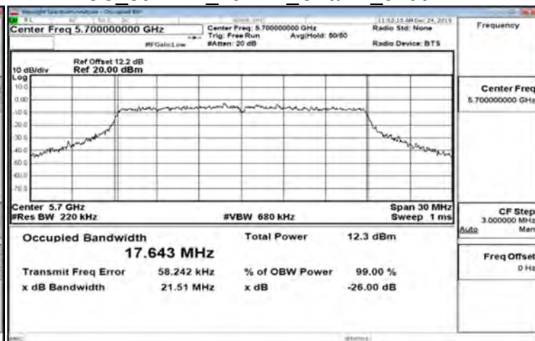
FCC 802.11n 20MHz_Chain1_5700MHz
