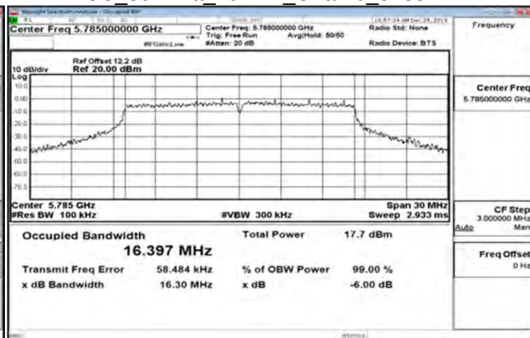
FCC 802.11a 20MHz_Chain0_5785MHz
