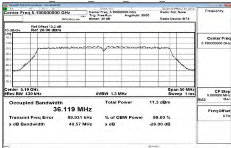
FCC 802.11n 40MHz_Chain1_5190MHz
