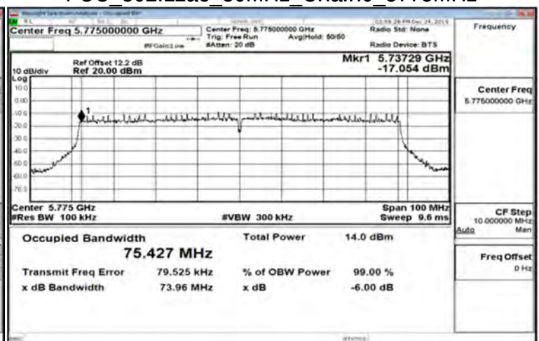
FCC 802.11ac 80MHz Chain0 5775MHz
