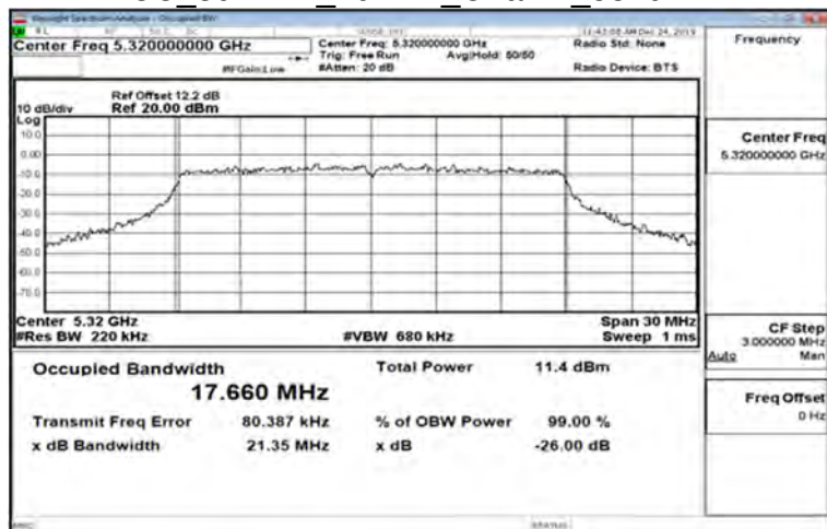
FCC 802.11n 20MHz_Chain1_5320MHz
