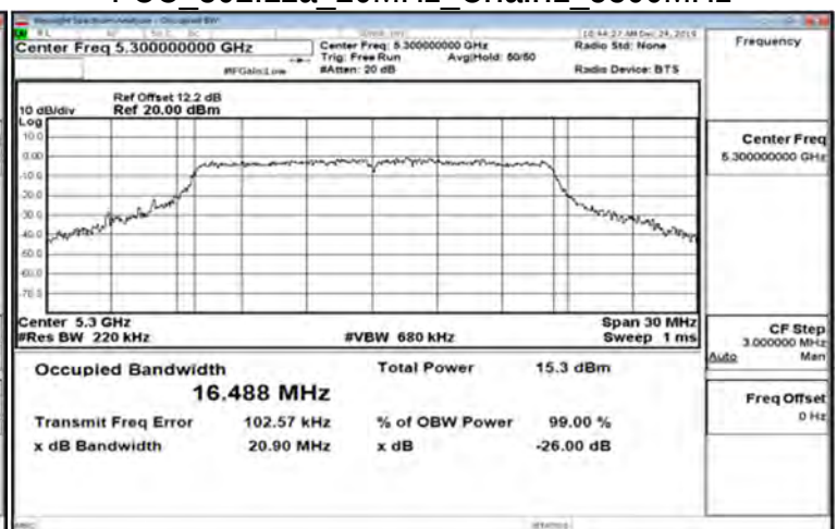
FCC 802.11a 20MHz_Chain1_5300MHz
