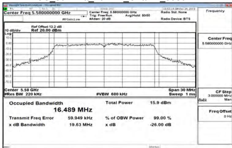
FCC 802.11a 20MHz_Chain1_5580MHz
