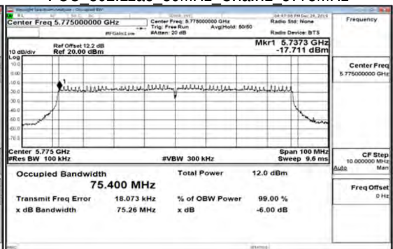
FCC 802.11ac 80MHz Chain1 5775MHz
