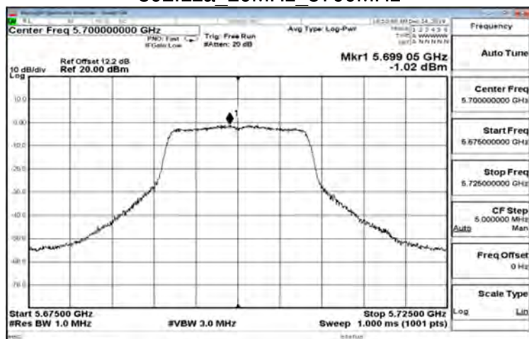
802.11a 20MHz 5700MHz
