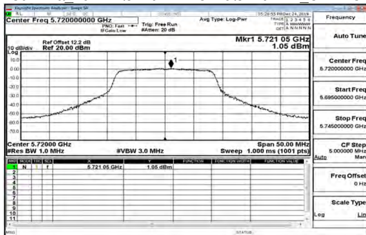
802.11a 20MHz\5720 MHz-5720\5720MHz UNII 3
