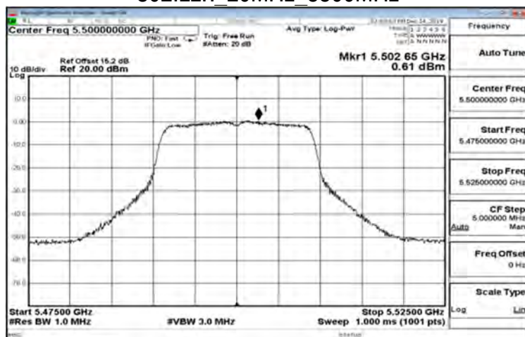
802.11n 20MHz 5500MHz
