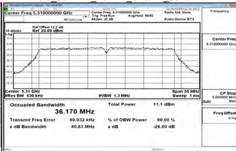
FCC 802.11n 40MHz_Chain1_5310MHz
