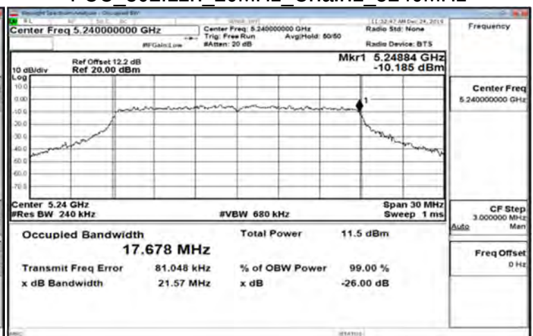
FCC 802.11n 20MHz_Chain1_5240MHz
