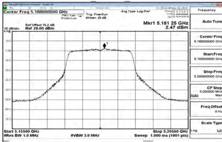
802.11n 20MHz 5180MHz
