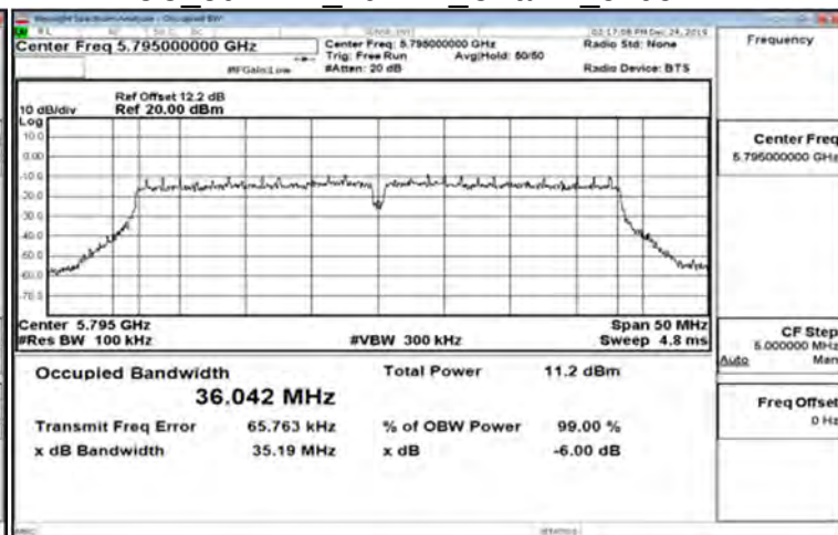
FCC 802.11n 40MHz_Chain1_5795MHz
