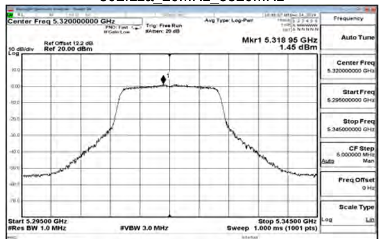
802.11a 20MHz 5320MHz
