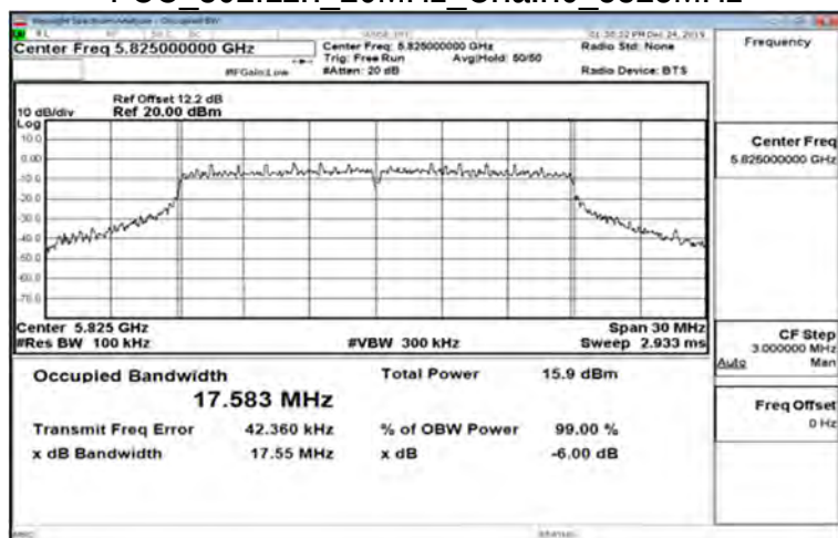
FCC 802.11n 20MHz_Chain0_5825MHz
