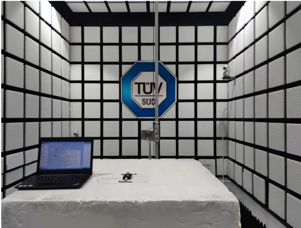
1GHz ~ 18GHz
