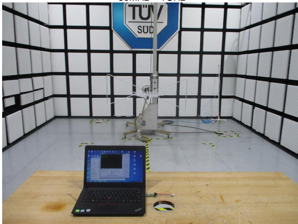
30MHz ~ 1GHz
