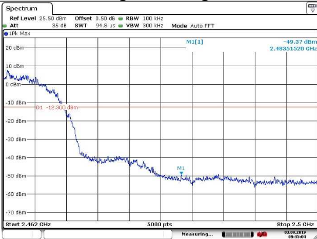
High band edge
