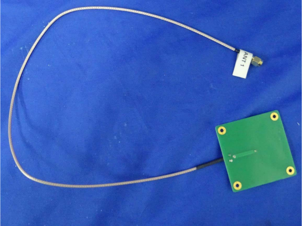
(37) EUT Photo _ANT 1
