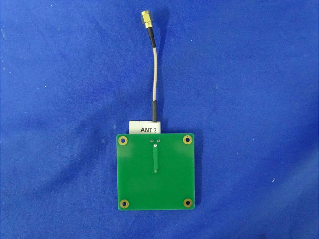
(16) EUT Photo _ANT 2
