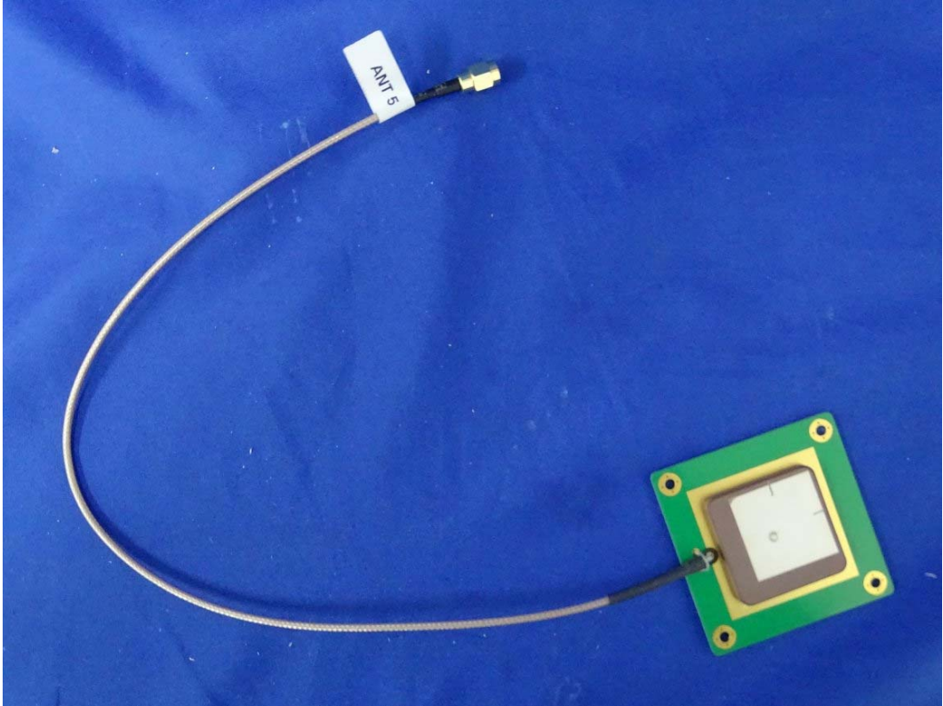
(21) EUT Photo _ANT 5
