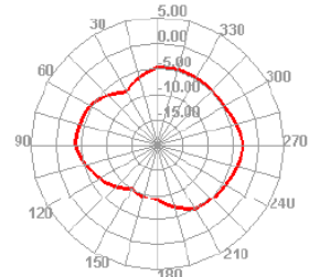
2480.000MHz E2
