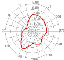
2480.000MHz E1
