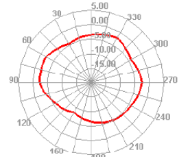
2440.000MHz E2
