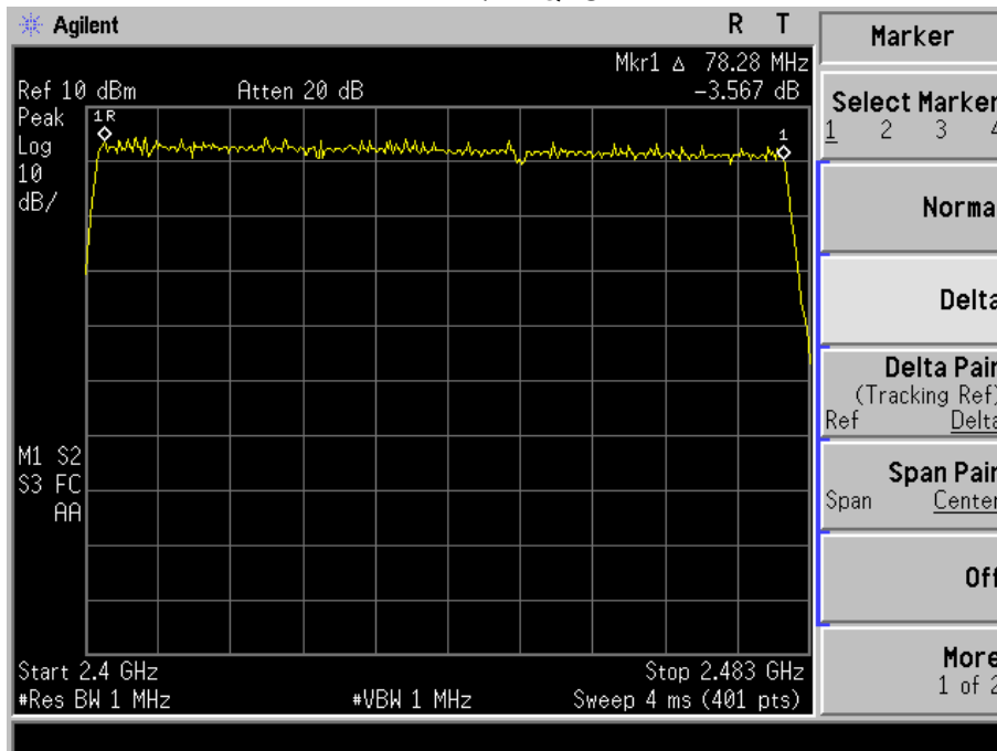
Pi/4 DQPSK
