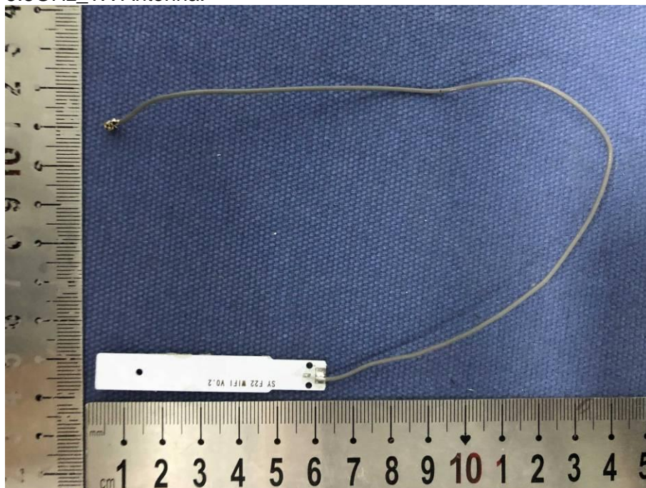
2.4GHz_RX Antenna:
