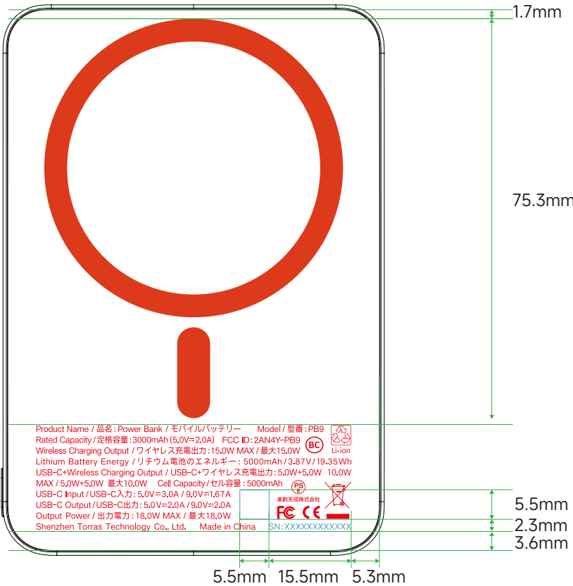
磁吸圈、铭牌左右居中
