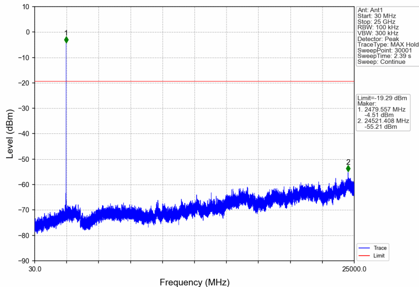
2M_HCH_2480MHz_Ant1_NTNV
