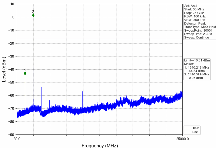
2M_HCH_2480MHz_DataRate=_Ant1_NTNV
