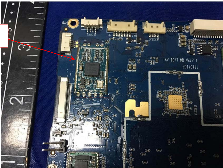
13.56MHz Module
