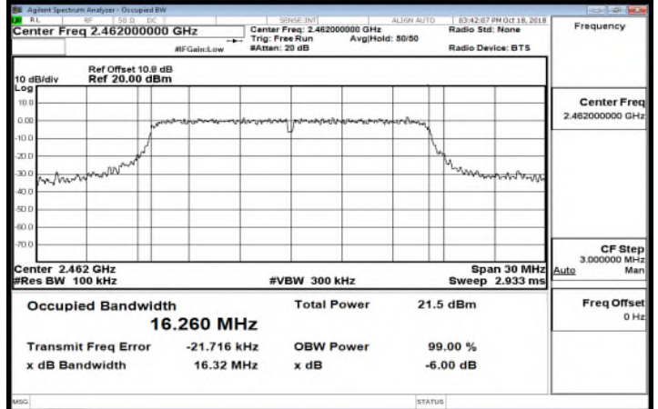
OBW 6dB_802.11g_20MHz_Chain0_2462MHz
