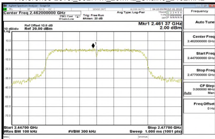
Reference Level_802.11n_20MHz_Chain0_2462MHz
