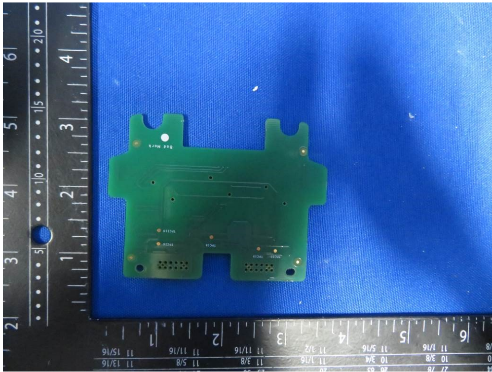
(31) EUT Photo
