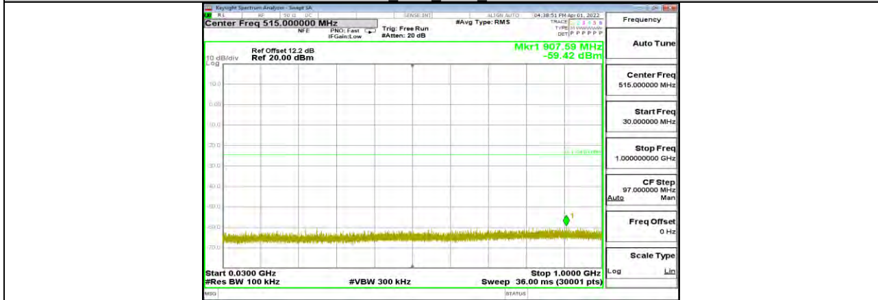
11N40SISO Ant1 2437 30~1000
