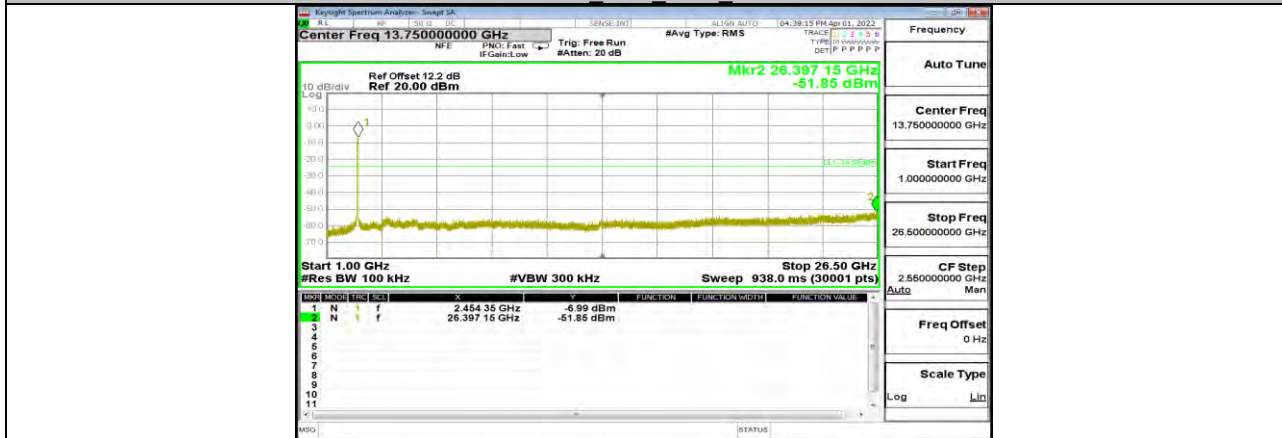
11N40SISO Ant1 2437 1000~26500
