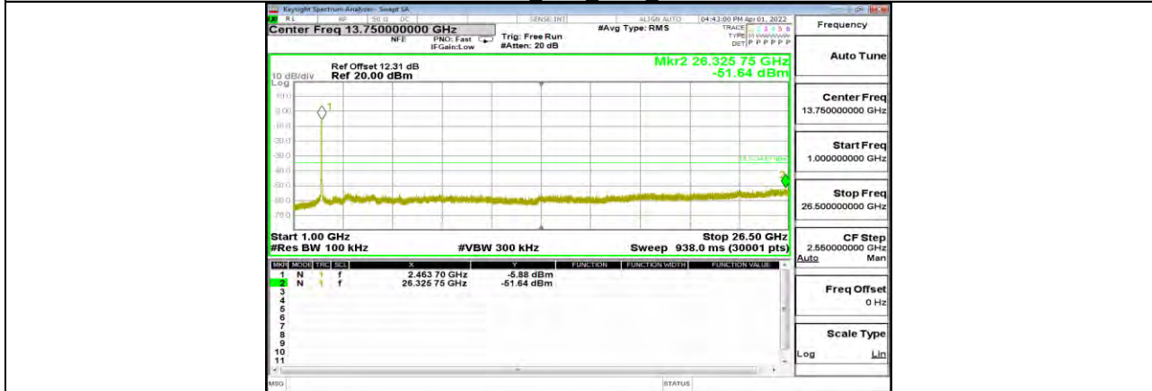
11N40SISO Ant1 2452 1000~26500
