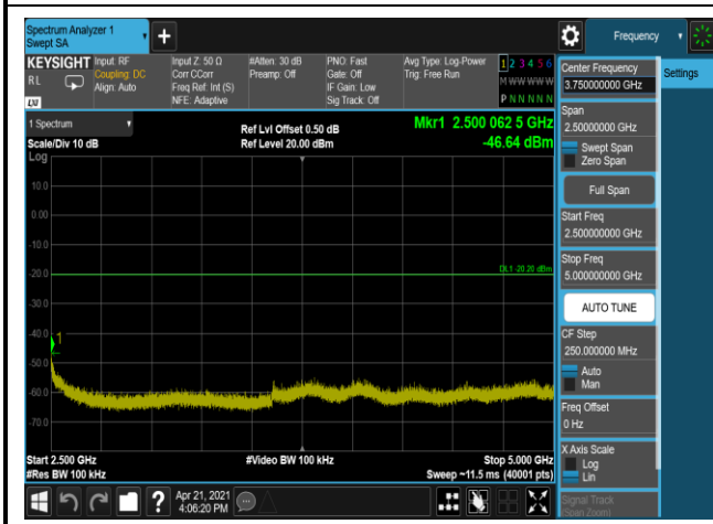
802.11n(HT40),2452MHz,Ant0,Plot 4,2500MHz~5000MHz
