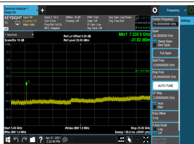
802.11b,2412MHz,Ant0,Plot 5,5000MHz~25000MHz
