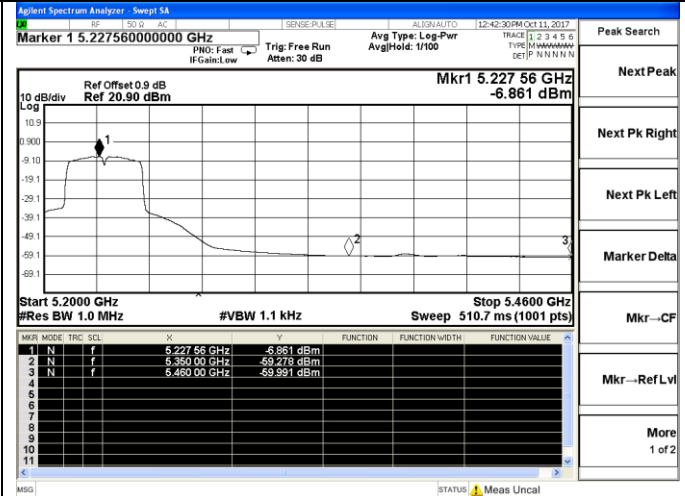
5230MHz (Average)
