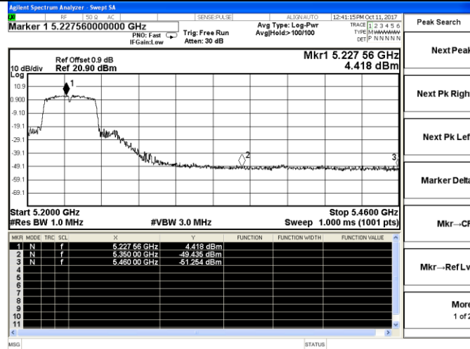
5230MHz (Peak)
