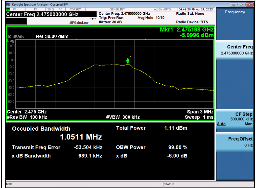
Test_Graph_2.4G_ANT1_2475_GFSK_DTSBW
