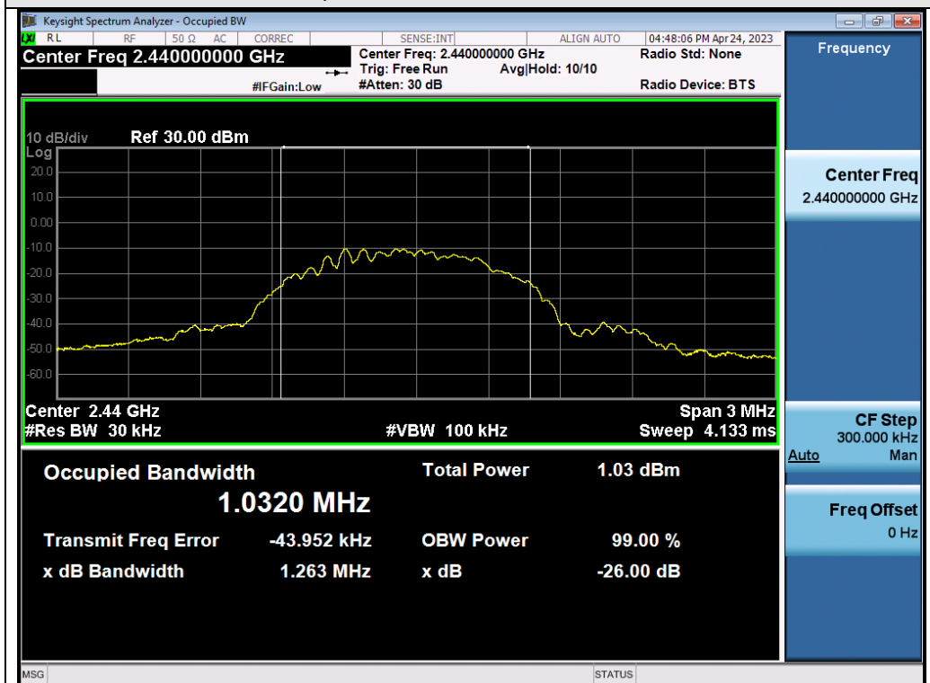
Test_Graph_2.4G_ANT1_2440_GFSK_OBW
