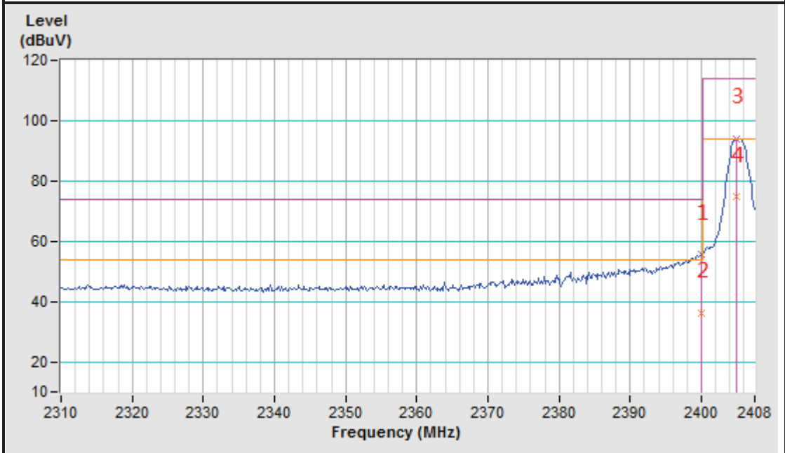
2405MHz Vertical
