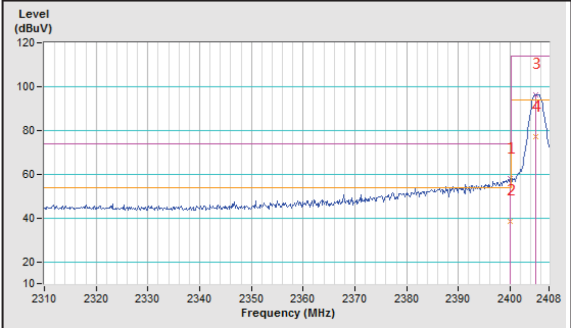
2405MHz Vertical
