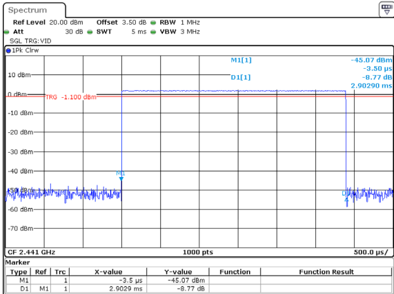
DH5_Hopping 2.903ms
