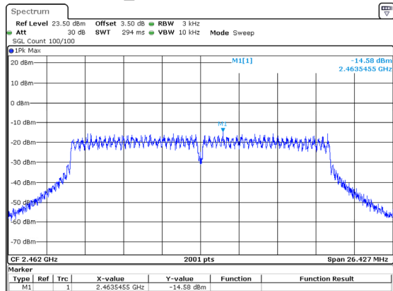
802.11n20_2462MHz -14.58dBm/3kHz
