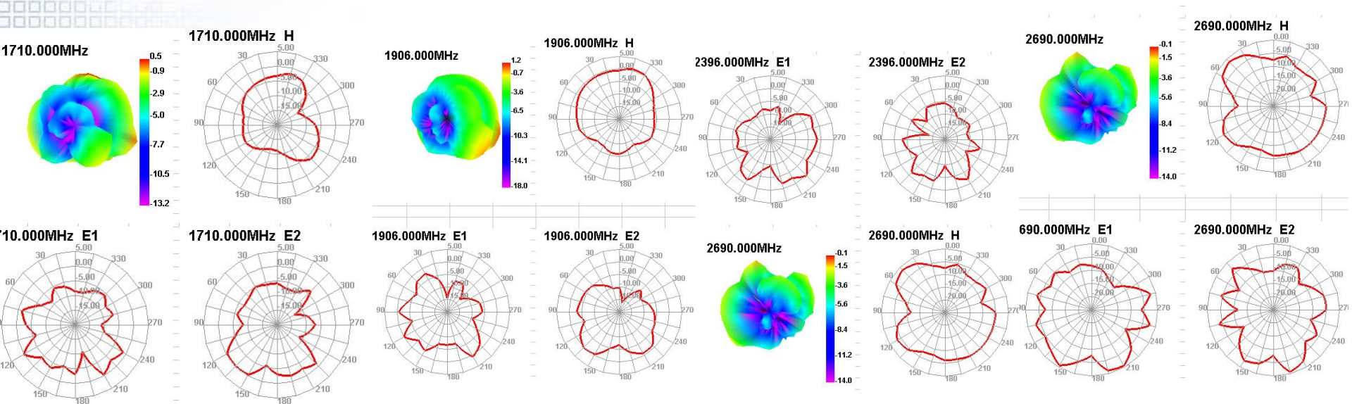
1710.00MHz - 2690.00MHz Gain
