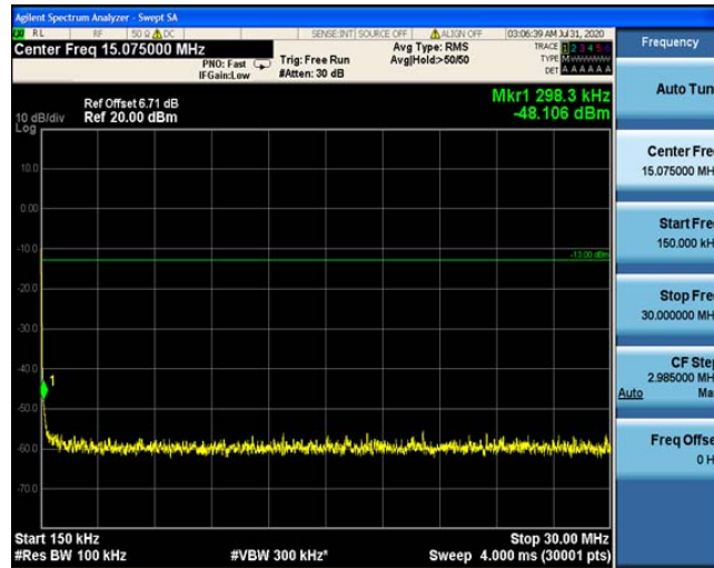
0.15~30MHz
