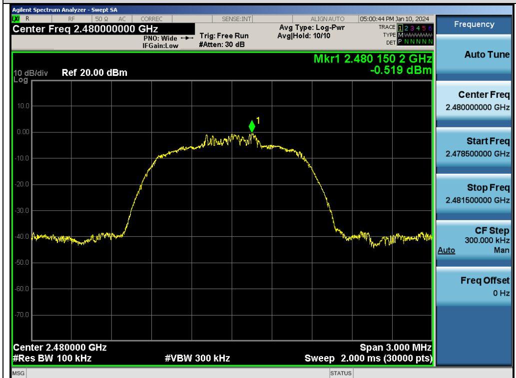
Test_Graph_EDR_ANT1_2480_2Mbps_Reference Level
