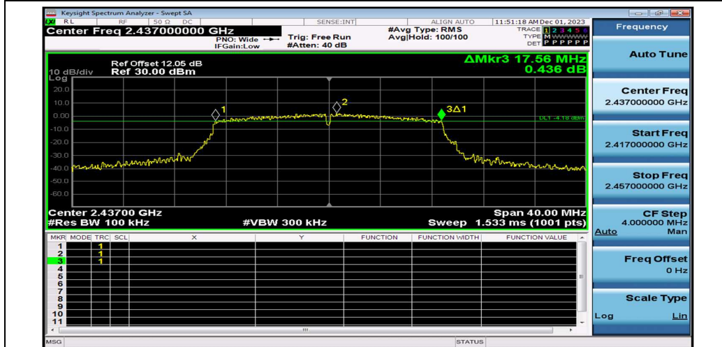
11N20SISO_Ant1_2437
