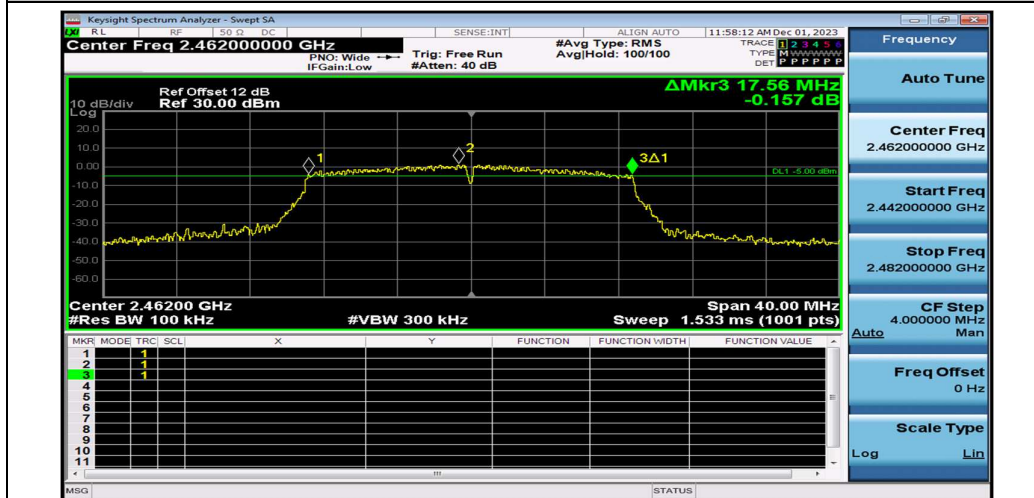
11N20SISO_Ant1_2462
